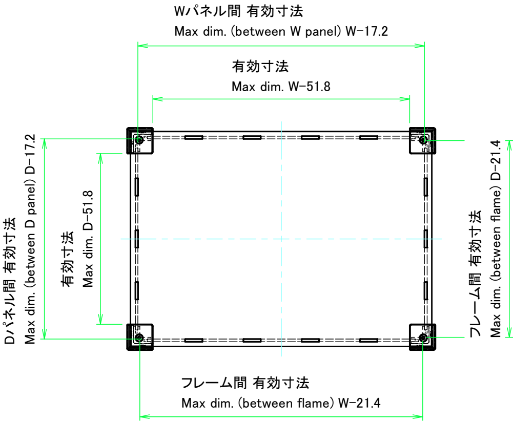
下カバー / Bottom cover
